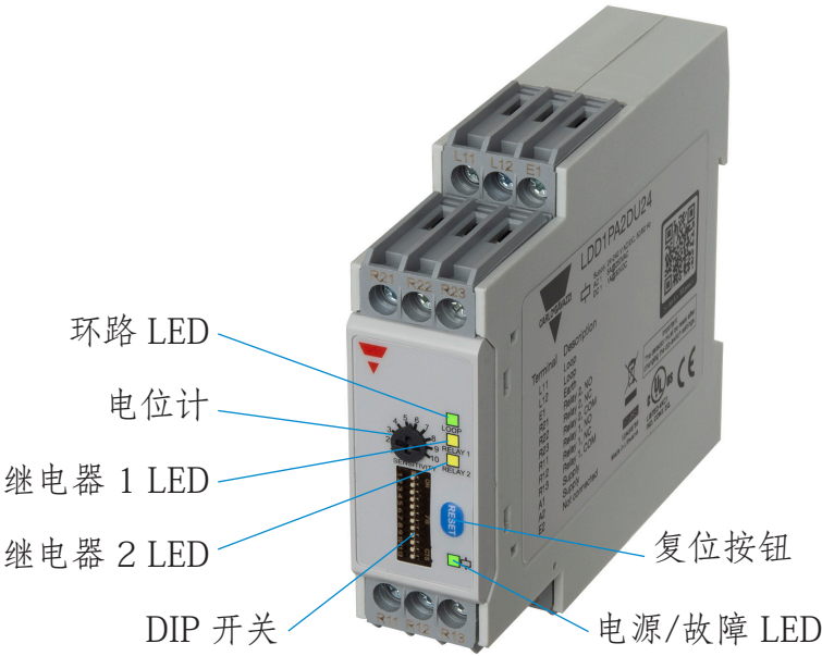
LDD1 单环路
